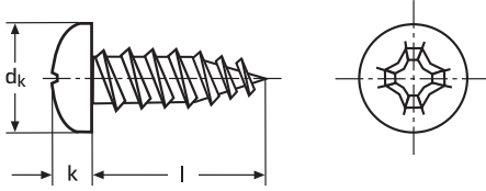
Form "C" mit Spitze
