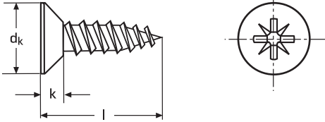
Form "C" mit Spitze
