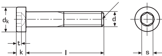
Kegelkuppe nach DIN 78
