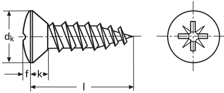
Form "C" mit Spitze
