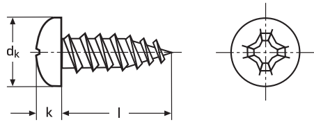
Form "C" mit Spitze
