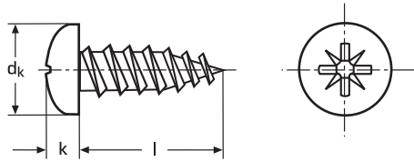
Form "C" mit Spitze
