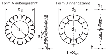
Form "A" außengezahnt Form "J" innengezahnt
