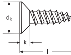
Form "C" mit Spitze
